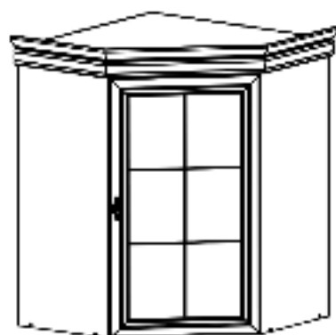
Kora KNN1
